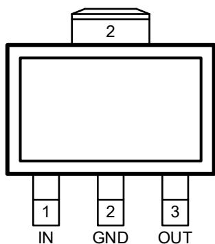
SOT-223 AxxG
