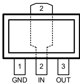
SOT-89-3L AxxP
