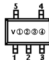
SOT-23-5L
