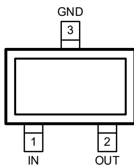
SOT-23-3L AxxMC
