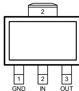
SOT-223 AxxGL
